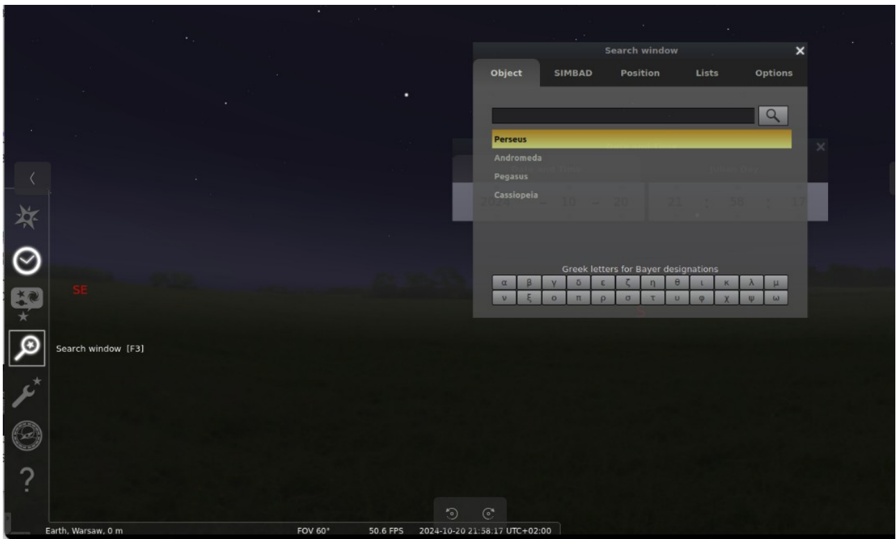
Rysunek 7. Zrzut ekranu z programu Stellarium.
