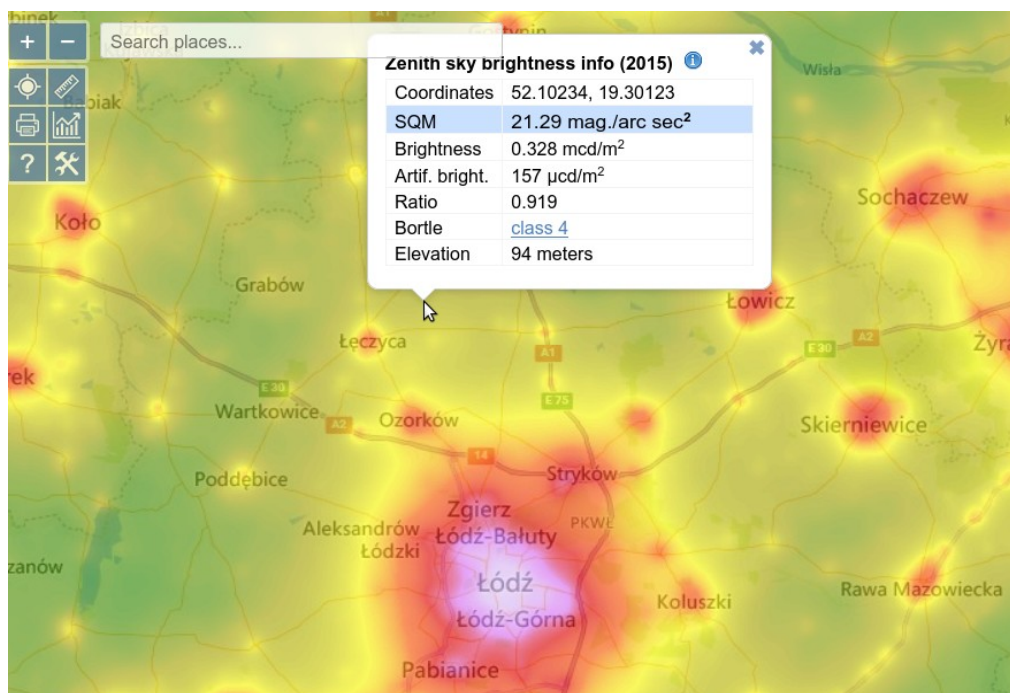
Rysunek 10. Wyznaczanie poziomu zanieczyszczenia światłem na mapie lightpollutionmap.info .
