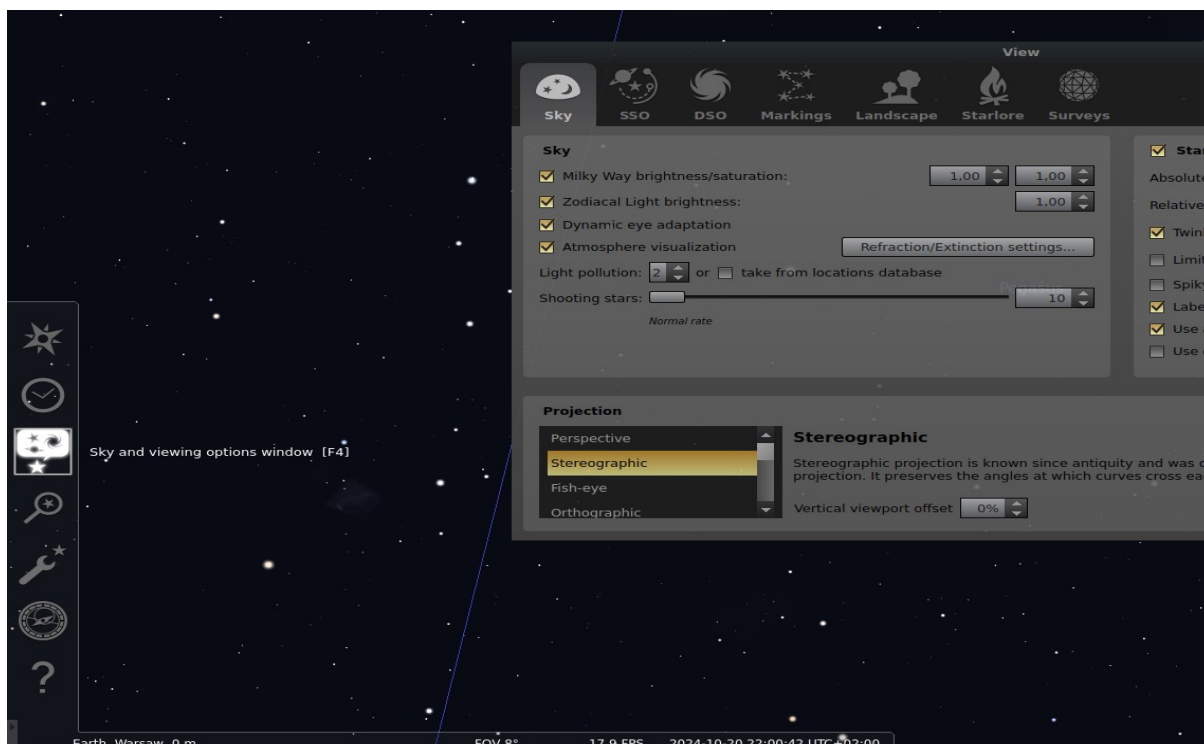
Rysunek 9. Zrzut ekranu z programu Stellarium.
