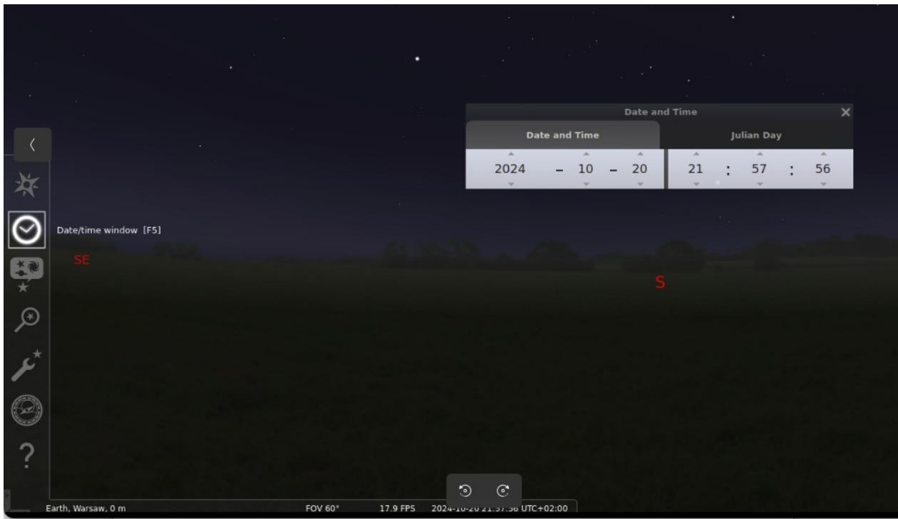
Rysunek 5. Zrzut ekranu z programu Stellarium.
