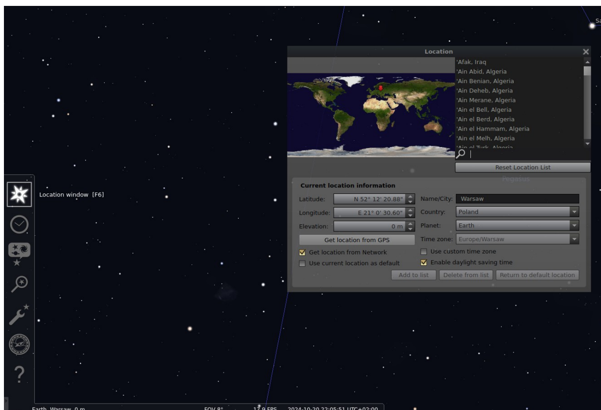
Rysunek 4. Zrzut ekranu z programu Stellarium.
